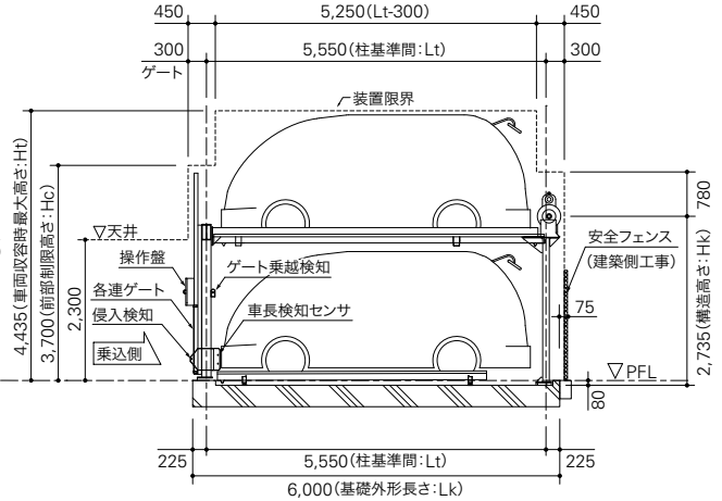
装置側面図
