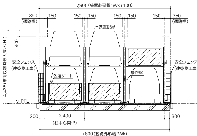
装置正面図
