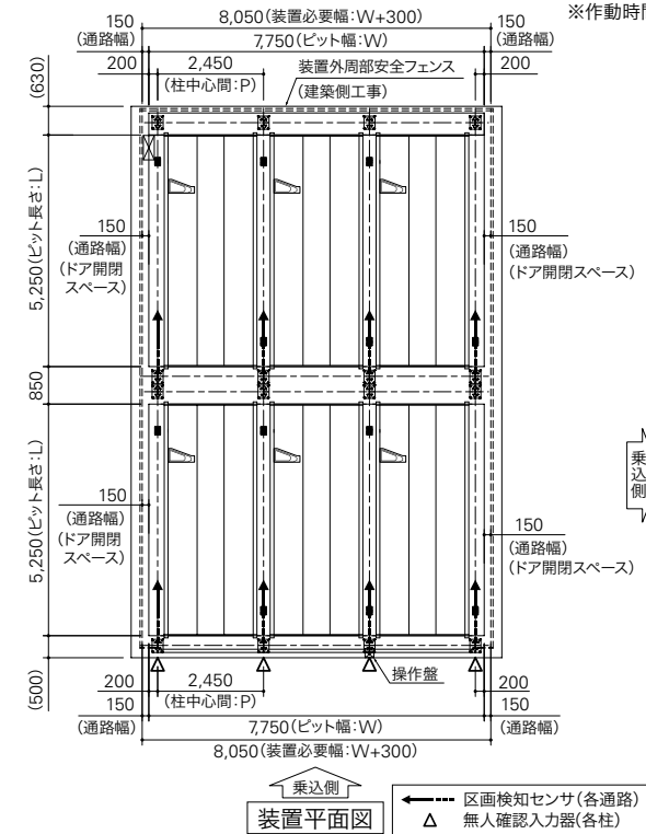
装置平面図
