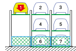
③ 1番下降
