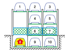
③ 8番上昇
