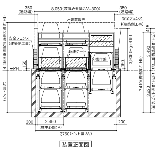
装置正面図
