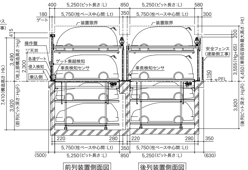
前列装置側面図
